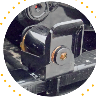
Roller for smoother container shift on the hook lift Rouleau de déplacement du conteneur vers le mécanisme
